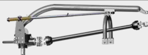
Level handle keeping the auger vertical position for digging and transport Рычаг для поддержания вертикальной стабильности буры в рабочем режиме
