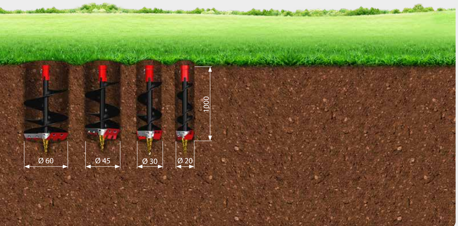
Replaceable knives and point Сменные ножи и долоты
