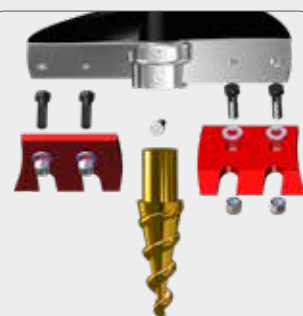
Replaceable knives and point Сменные ножи и долоты
